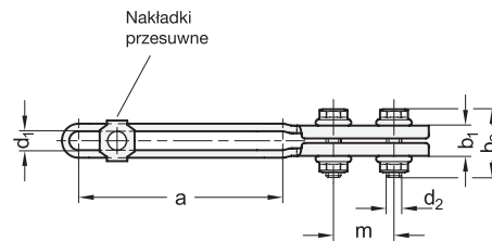
Przykład montażu
